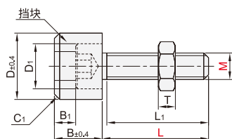
内六角圆柱挡块 51/52
