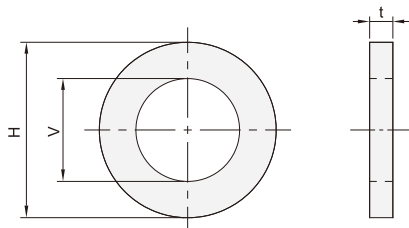
平垫圈型
