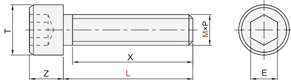
内六角圆柱头螺钉 YAB01/02/03
