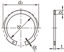
挡圈尺寸
