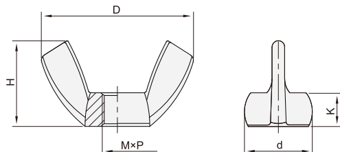
蝶型螺母 YBK01/02
