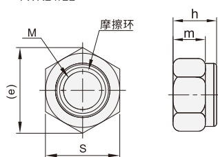
非金属嵌件六角锁紧螺母 YWR21/22
