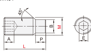
凸头型 YWK31
