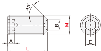
凹头型 YWK11/12
