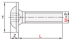
内六角平头带垫螺钉 YWD06/07
