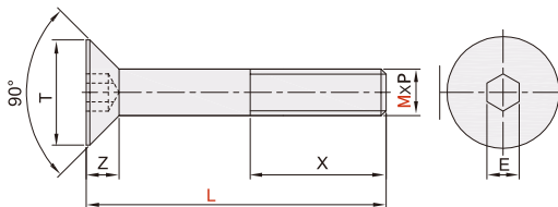
内六角沉头螺钉 YWH01 YWH02
