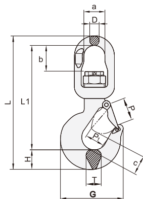
旋转吊钩
