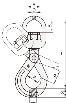
80级旋转自锁钩
