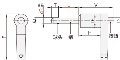
顶出L型 YAA12
