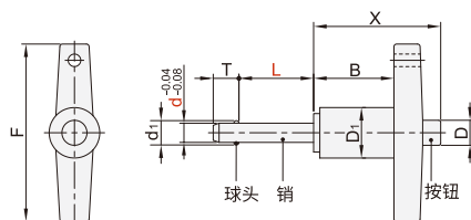
顶出T型 ZAA11
