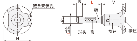
顶出防护型 YAA02
