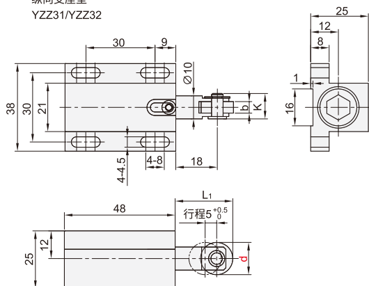
纵向支座型 YZZ31/YZZ32
