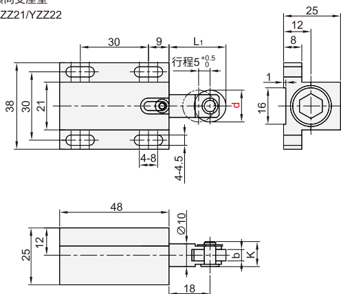
■横向支座型
