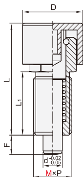
无锁紧螺帽 YZB51/YZB52
