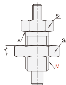
带锁紧螺帽 YZB31/YZB32
