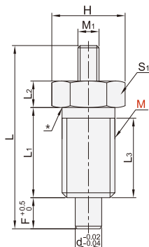
无锁紧螺帽 YZB21
