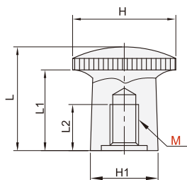
压入式专用旋钮 YZU73
