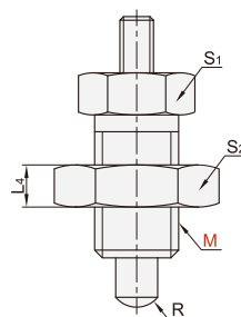
带锁紧螺帽 YZB11/YZB12
