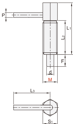
无锁紧螺帽 YZU51/YZU52
