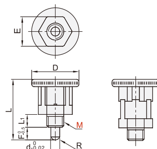
自锁型 YZU11/YZU12
