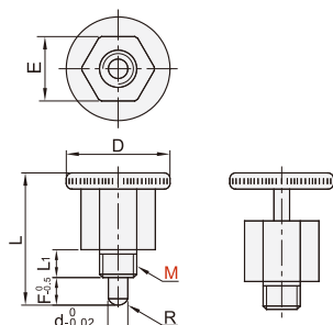
复位型 YZU01/YZU02
