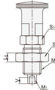
带锁紧螺帽 YZT13/YZT14
