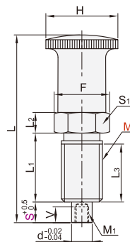
无锁紧螺帽 YZT01/YZT02
