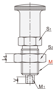
带锁紧螺帽 YZT03/YZT04
