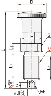
无锁紧螺帽 YZT11/YZT12
