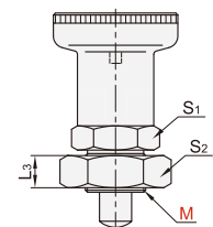
自锁型 带锁紧螺帽 YZY34
