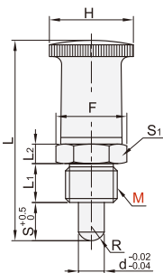
复位型 无锁紧螺帽 YZY23
