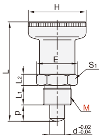
复位型 无锁紧螺帽 YZY23
