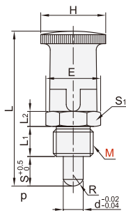
自锁型 无锁紧螺帽 YZY33
