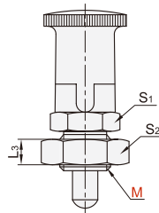
自锁型 带锁紧螺帽 YZY34
