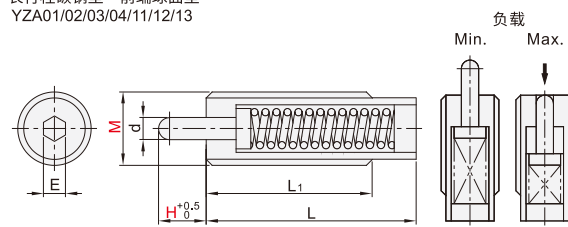
长行程碳钢型 · 前端球面型 YZA01/02/03/04/11/12/13
