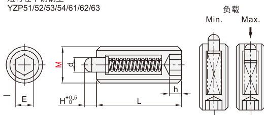
短行程不锈钢型 YZP51/52/53/54/61/62/63
