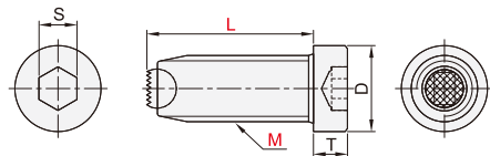
齿型 YZX02
