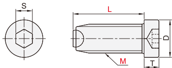
齿型 YZX02
