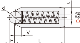
重载 YZL32
