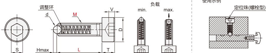
内六角螺栓型 YZK01/03/02/04
