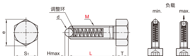
外六角螺栓型 YZK11/13/12/14
