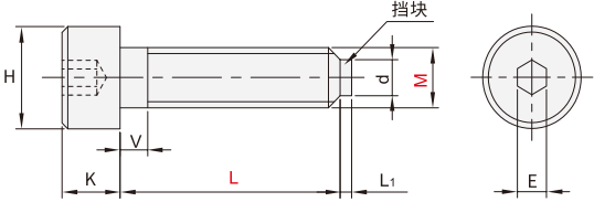
直杆型 YTC01/02/11/12
