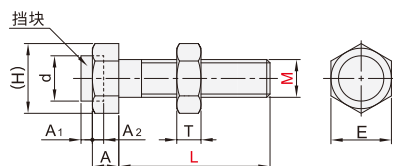
标准型 / 平头型 YTB11 / 12 / 21 / 22 / 31 32 / 42
