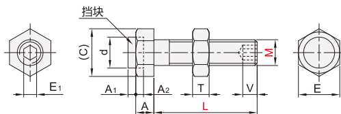
内六角孔型 / 平头型 YTB61/62/71/72
