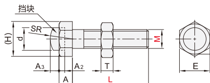
标准型 / SR型 YTB51 / 52
