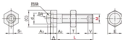
内六角孔型 / SR型 YTB81/82
