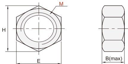
六角螺母型
