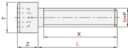
内六角圆柱头螺钉 YAB01/02/03
