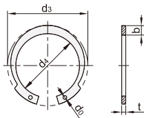
挡圈尺寸
