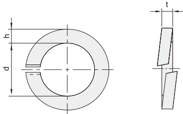
■GB/T93-1987
