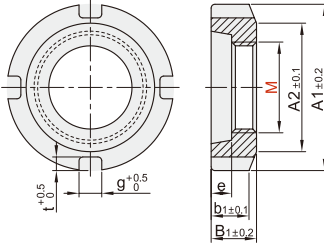
凹螺母
