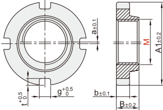
凸螺母
