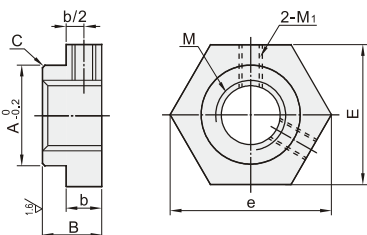
六角型 紧定螺钉型 GYAJ41/46/51/56/61
