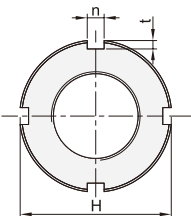
小圆螺母 GYBP01
