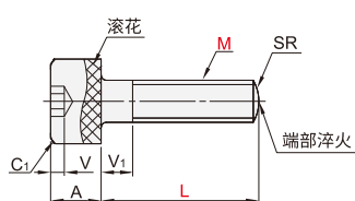
■六角螺栓型
