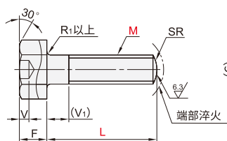
六角螺栓型
