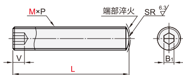
■紧定螺钉尺寸
