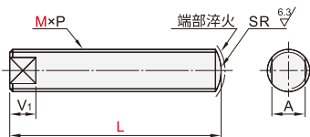
带扳手槽型
