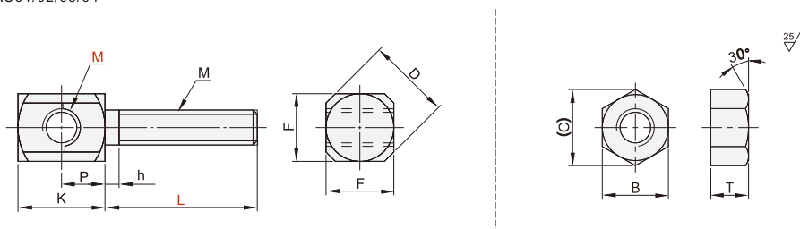
螺栓型 YAU01/02/03/04
