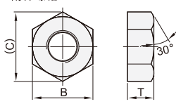
附件螺母
