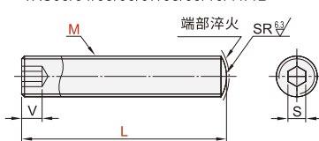
内六角孔型
