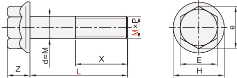
六角法兰面螺栓 YAH01 YAH02
