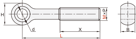
活节螺栓 YAH03
