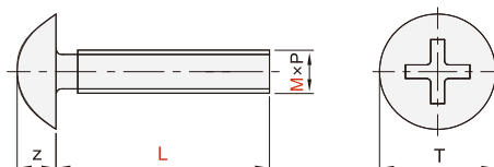
十字槽大扁头螺钉 YWL06
