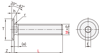
超薄头型 YWN03
