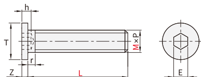
内六角超短头螺钉 YWN01/02
