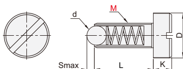
薄头螺栓型·金属球头 YZX21/YZX22
