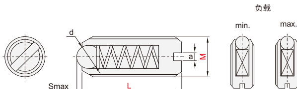
无防松型·树脂球头 YZJ03/YZJ06
