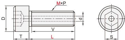
内六角圆柱头型 YWK21
