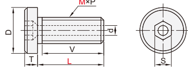
内六角薄圆柱头型 YWK22
