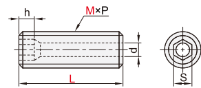
内六角紧定螺钉型 YWK25
