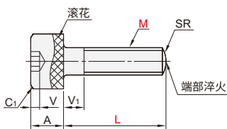
■六角螺栓型
