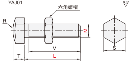
限位块
