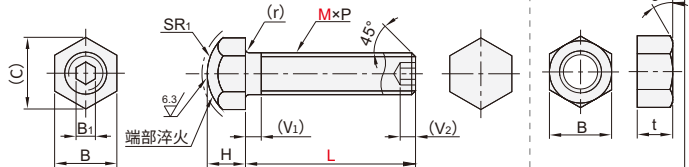
圆头内六角孔型 YAD55/56/57/58/59
