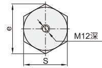
安装面尺寸
