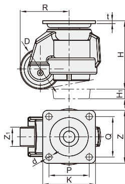
平底活动型 WKJ11
