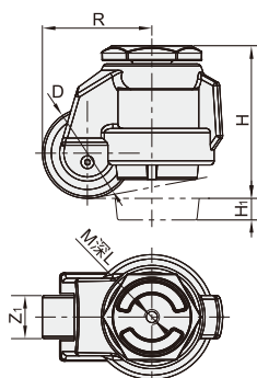
丝杆活动型 WKJ02
