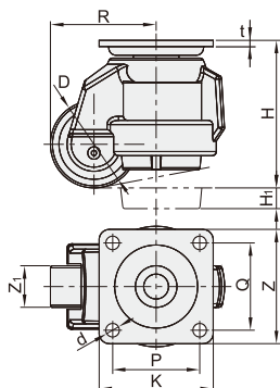
平底活动型 WKJ01
