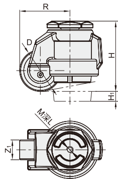
丝杆活动型 WKJ22
