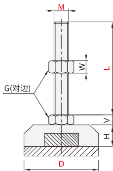
碳钢+橡胶底座型 WBM31
