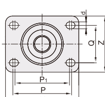
安装面 WKG71-D75
