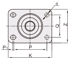
安装面 WKG01
