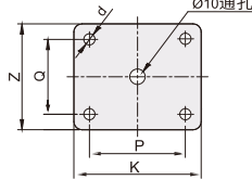
安装面 D75/75A
