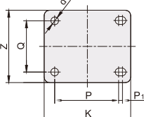
安装面 D50
