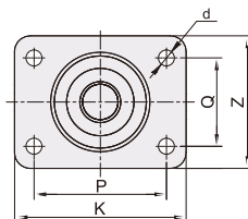
安装面 WKG71-D75A/D75B
