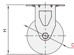
固定型 WHH21
