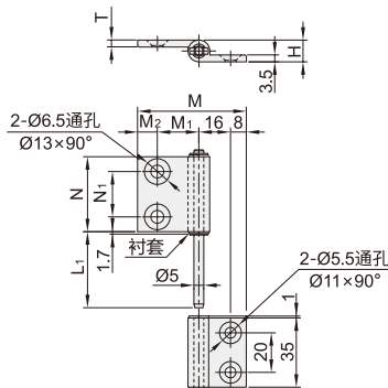
左右偏置锥孔型 VKF55/56
