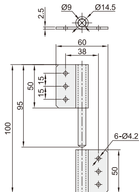
圆孔型 VKF41/42
